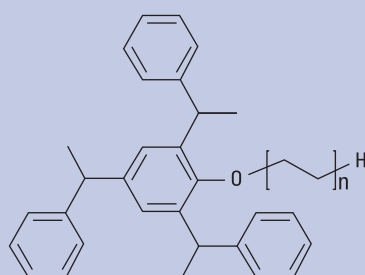
Общая формула продуктов группы Emulsogen® TS. Доступны продукты со степенью этоксилирования от 16 до 54.
