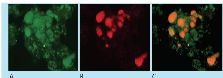
Рис. 1. Эти фотографии одной и той же дрейфующей частицы были сделаны электронным микроскопом: А - дрейфующая частица биомассы зеленая для всех бактериальных типов. В - показывает ту же самую частицу с красными пятнами, характерными для окисляющих аммиак бактерий. С - показывает совмещение этих двух картин, показывая пространственное распределение нитрификаторов в пределах одной хлопьеобразующей частицы.
