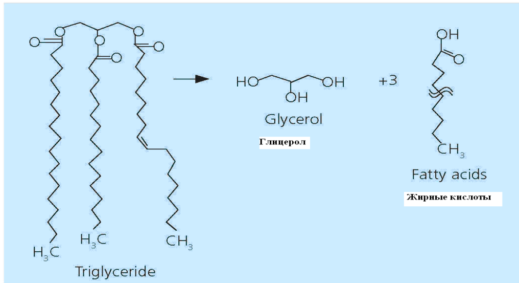
Рис. 1. Структура триглицерида.
