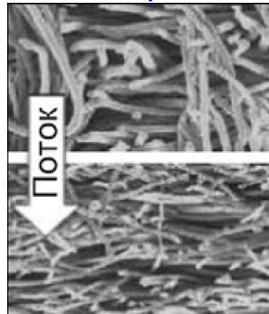
Рис. 1. Структура материала фильтра ДуоФЛО.
